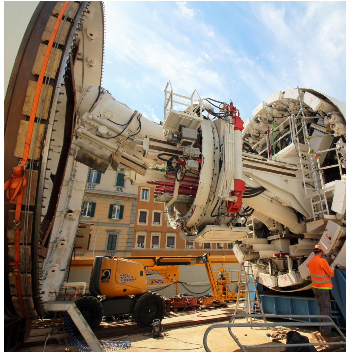
Varo della TBM - Talpa meccanica per lo scavo delle gallerie
