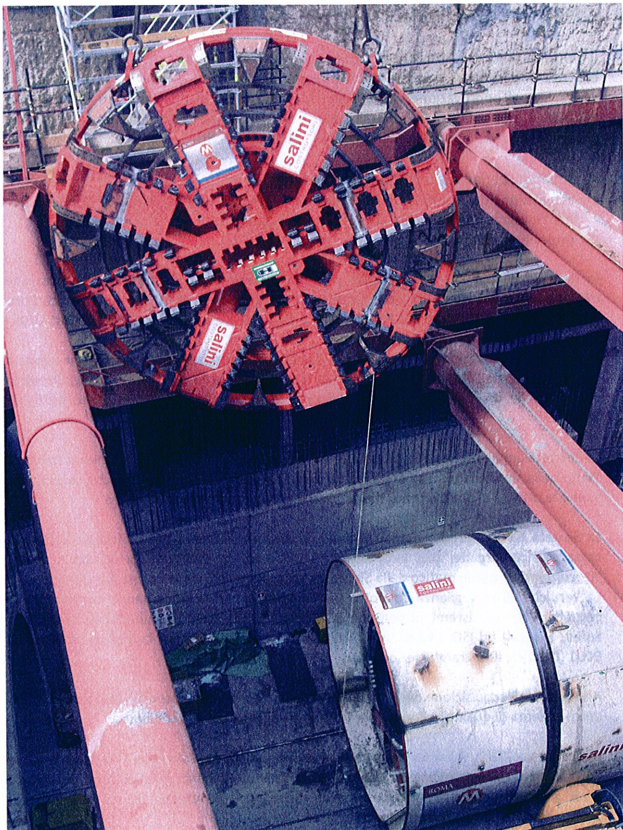
Italia, Metro B1 Roma
